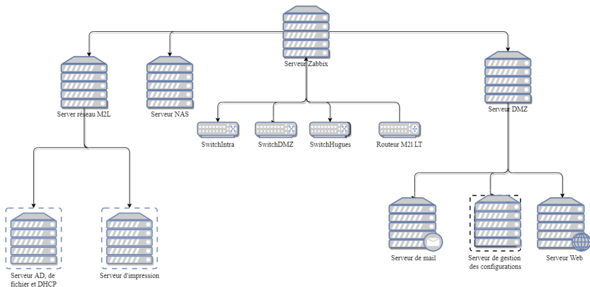
Schéma contextualisé de monitoring de l'infrastructure M2L
